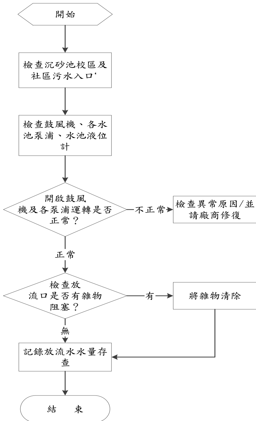
圖 116 生活污水處理廠設備維護作業流程圖
